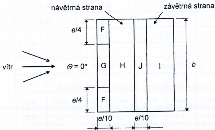
(b) směr větru \theta = 0^\circ
