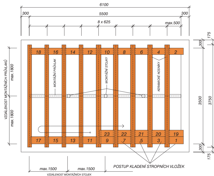
Obr. 1 Schéma montáže stropu (příklad)
