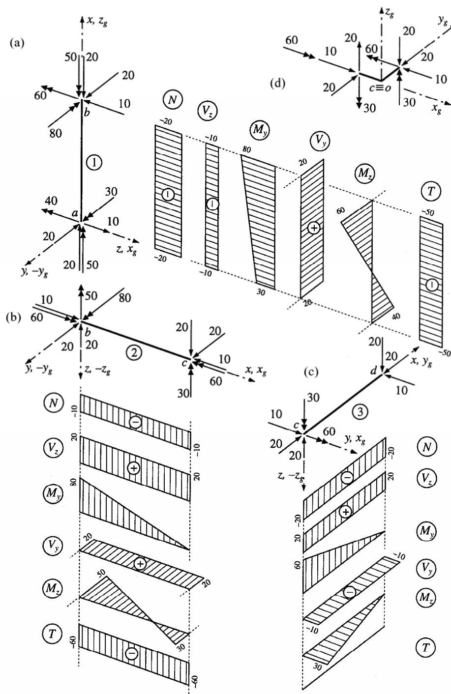
Obr. 4.10: Průběhy složek vnitřních sil na jednotlivých prutech nosníku v lokálních souřadnicových soustavách
