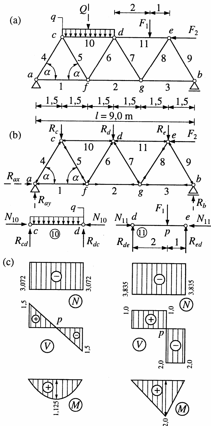
Obr. 3.15: Prutová soustava s mimostýčným zatížením
