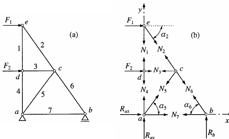
Obr. 3.6: Uvolněné styčnický prutové soustavy
